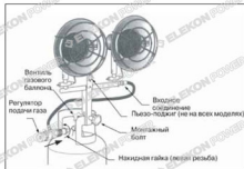
Рис.3. Внешний вид нагревателя. Звездочкой обозначены элементы, присутствующие у моделей с пьезо-поджигом.
