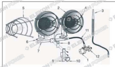
рис.1. Названия частей нагревателя
